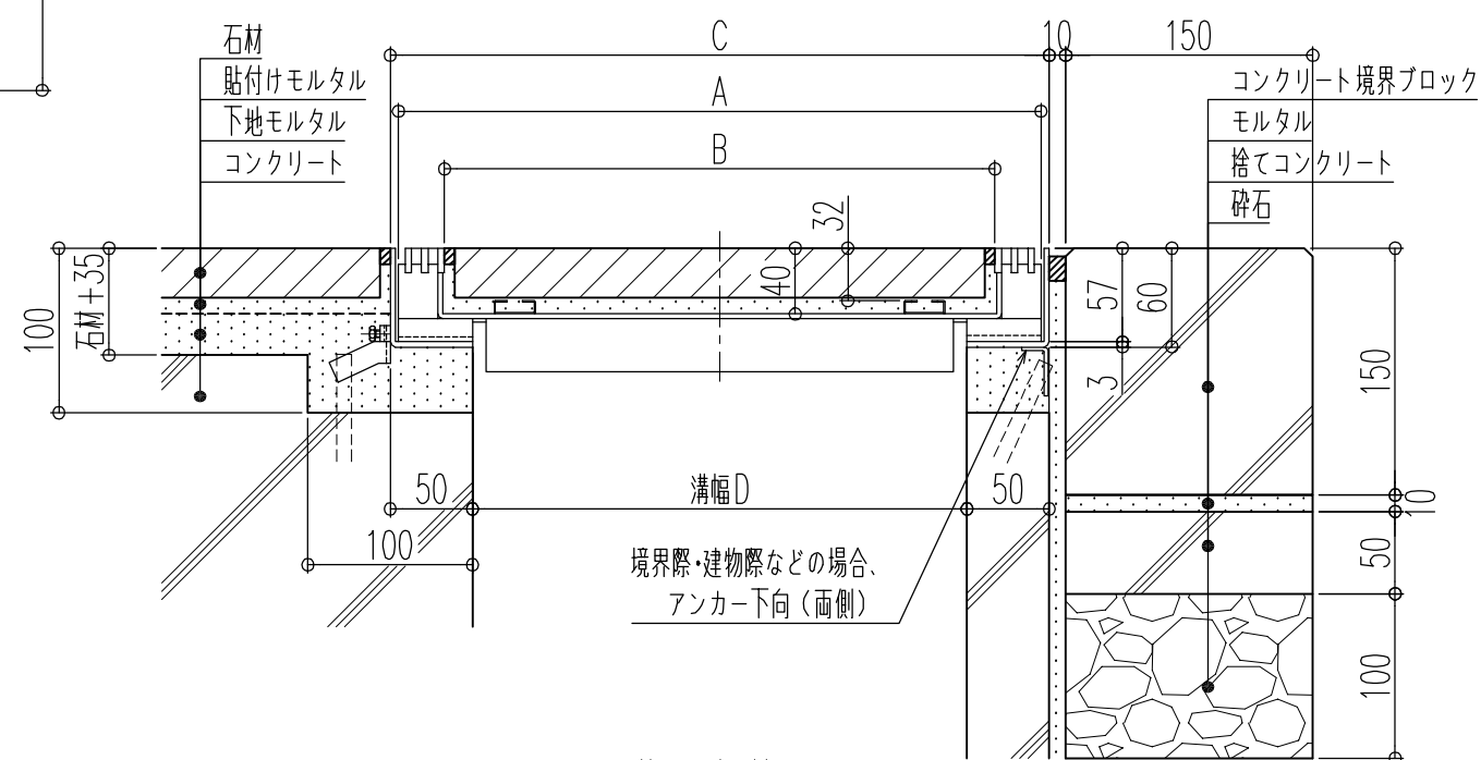
施工参考図
